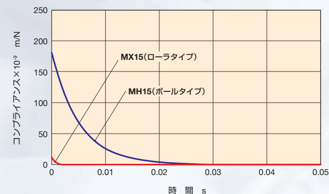
下方加振時の振動減衰曲線(片振幅)
