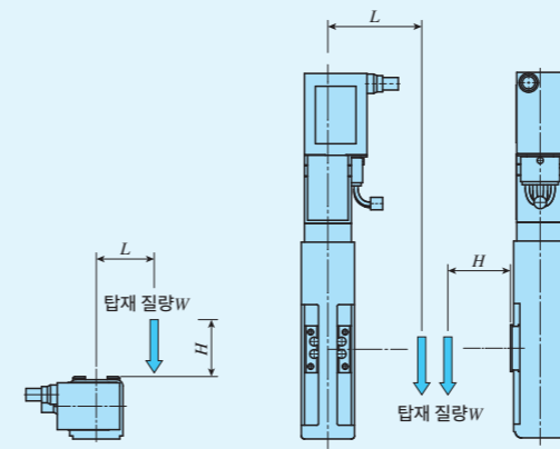
탑재 질량의 중심 위치 (수평 방향)
