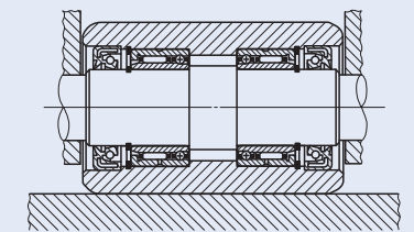
図 1 取付例
