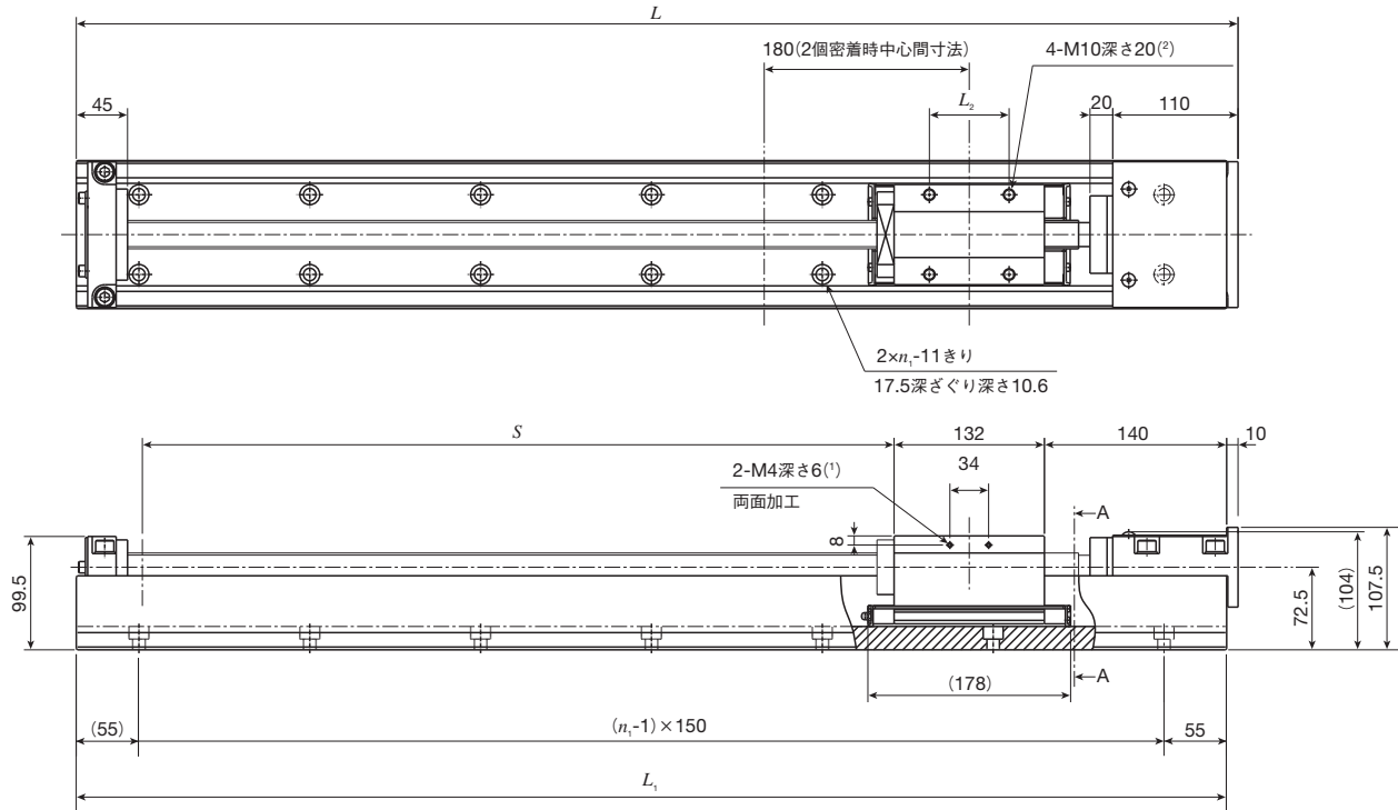
A-A 断面寸法
