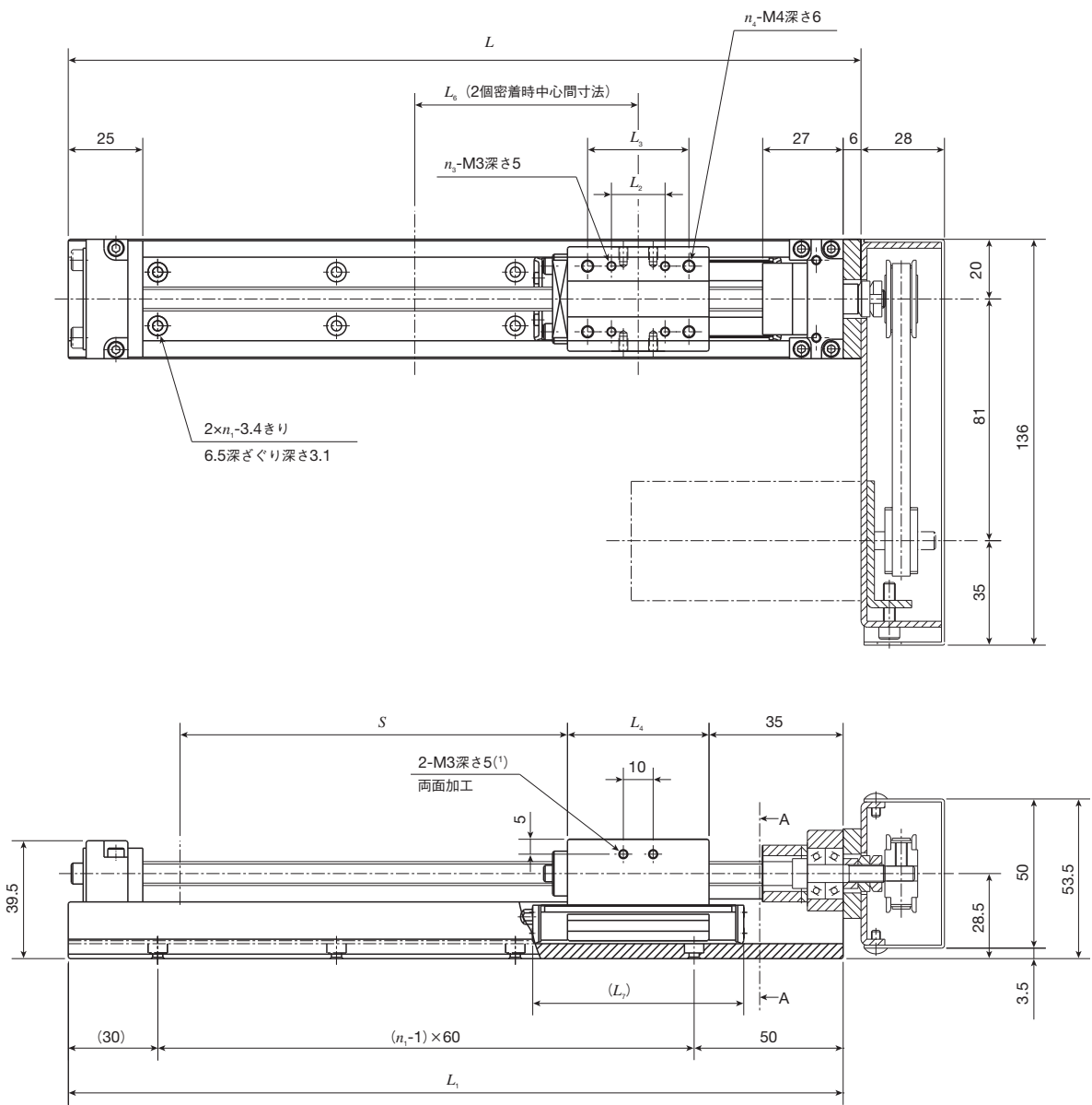
A-A 断面寸法
