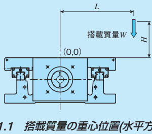
図1.1 搭載質量の重心位置(水平方向)
