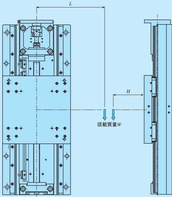
図1.2 搭載質量の重心位置(垂直方向)
