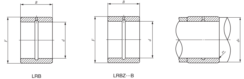
組合せ軸受
