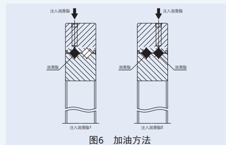
图6 加油方法
