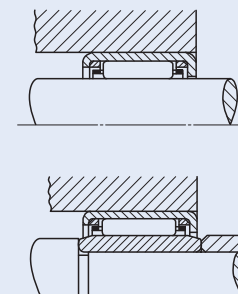
図2 取付例
