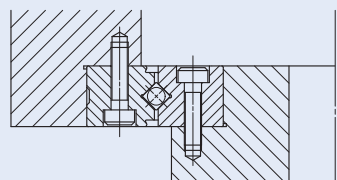
図5 高剛性取付穴付きクロスローラベアリングVのハウジングに取り付ける例
