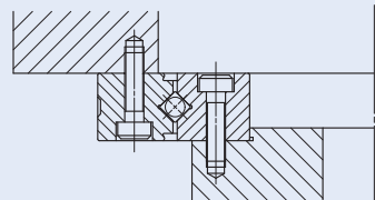
図3 高剛性取付穴付きクロスローラベアリングVの直接相手面に取り付ける例
