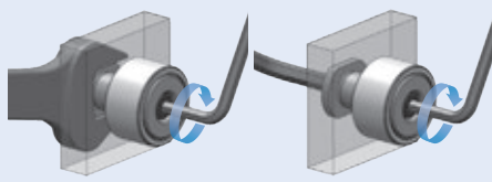
図3.2 スパナでフランジナットを回り止めする場合
