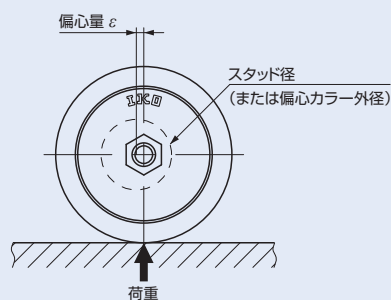
図5 偏心スタッドカムフォロア及び偏心カラー付きカムフォロアの調整の基準位置
