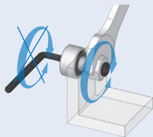
図3.1 取付方法
