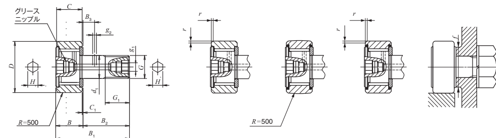
CFKR...VR 外輪外径 D 30~90mm
