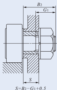
図 8 偏心カラー付きカムフォロアの取付穴の長さ
