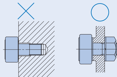
図4 取付方法
